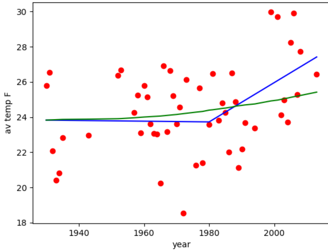
kuij 1980 vs co2
