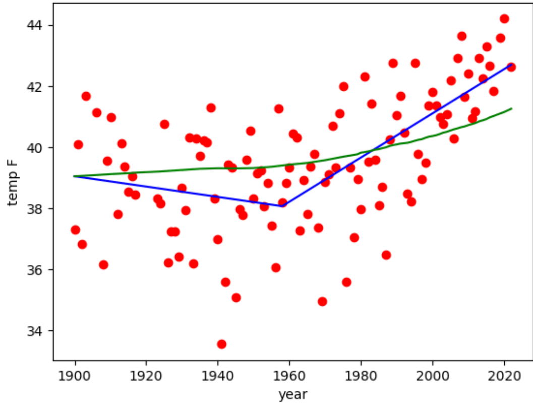
volga/oka 1958 tavmean vs co2
