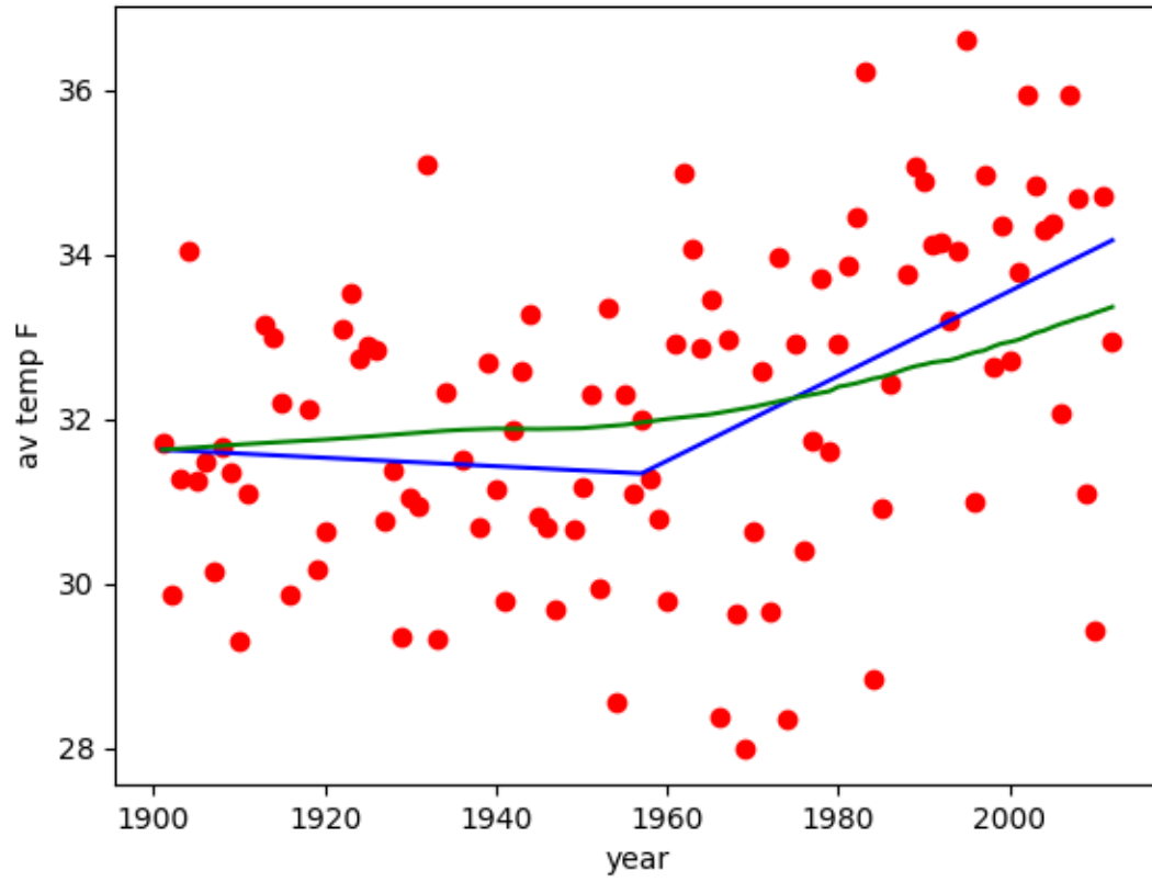
Tomsk 1957 vs CO2
