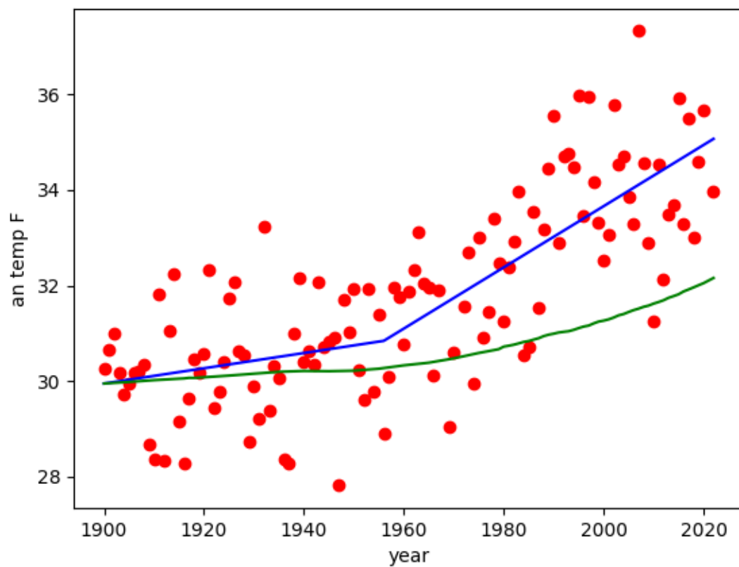
Irkutsk 1956 vs. CO2
