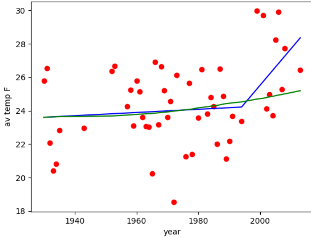
kuij 1993 vs co2
