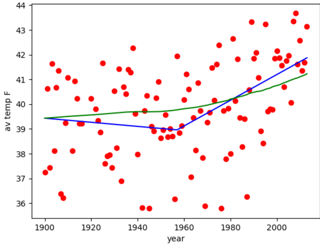
elatma 1957 vs. CO2
