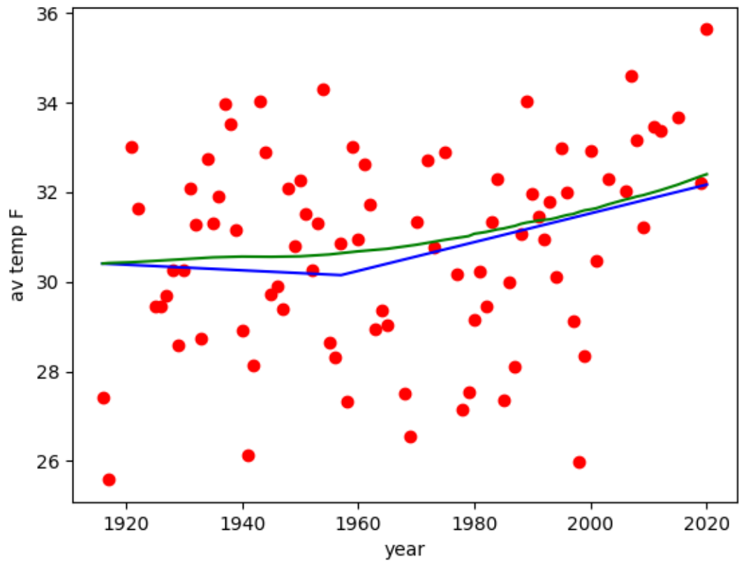
kanin nos 1957 vs. CO2
